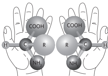
Рис. 1.2. Молекулы-стереоизомеры
