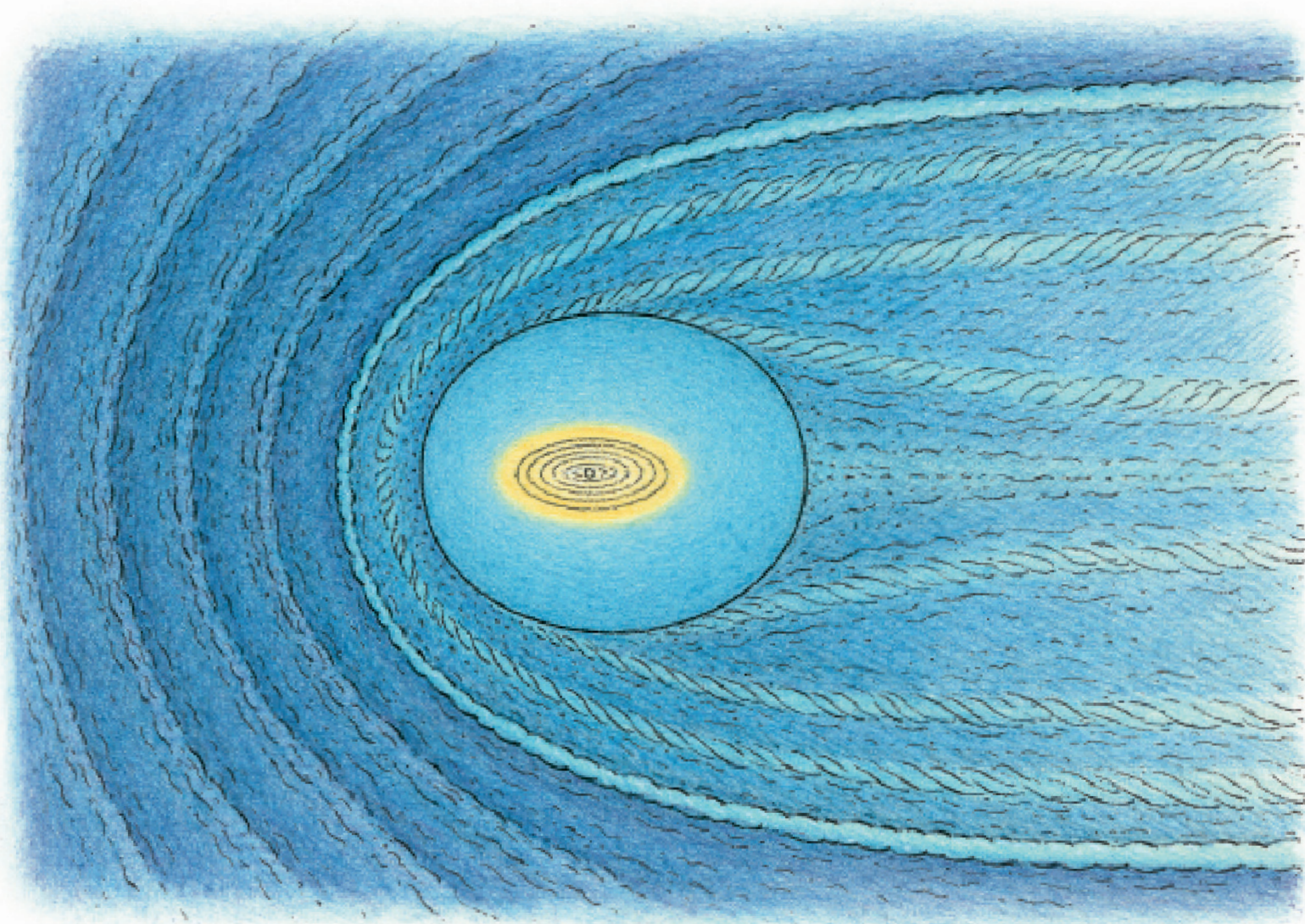
Наша Солнечная система похожа на огромный пузырь, плавающий в космическом пространстве. В его центре расположено Солнце, а его стенки — это гелиопауза.
