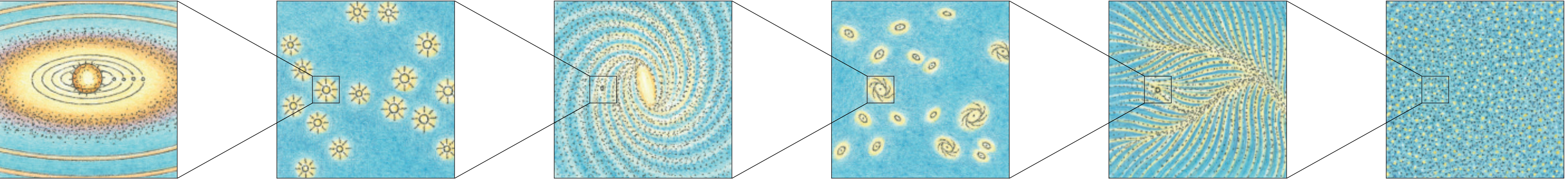
Солнце — центр Солнечной системы, одна из десятков звезд в... нашей окрестности, которая представляет собой крошечную часть... рукава Ориона — одного из рукавов спиральной структуры Млечного Пути, одной из нескольких десятков галактик в группе, которая входит в... сверхскопление Ланиакея, в котором есть еще около 100 000 галактик... что составляет меньше одной миллионной от числа галактик в известной Вселенной.
